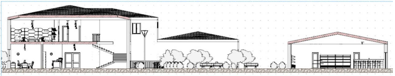
Sezione A-A'
